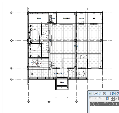
【1F 平面図】
