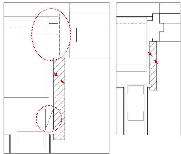
【1/30 ( 断面形状 2D 作図する )】
