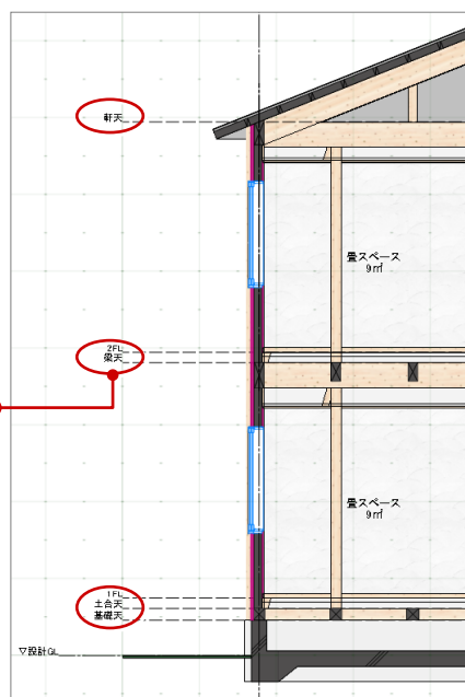
【断面ビュー】
