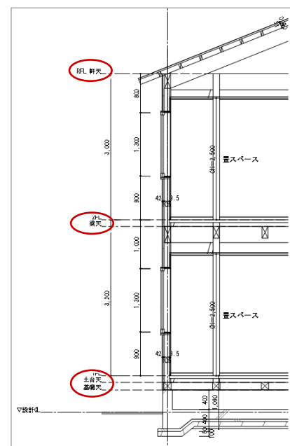
【矩計図】
