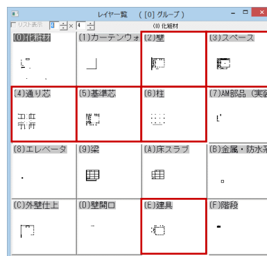
【平面図のレイヤー一覧】
