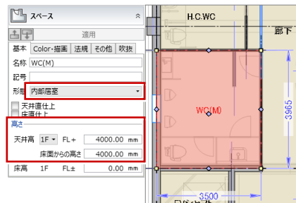
【スペース配置後のプロパティ】
