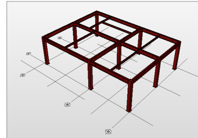
【(1 階) 柱・梁以外の部材を OFF にした例】
