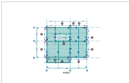
【3階 梁伏図】
