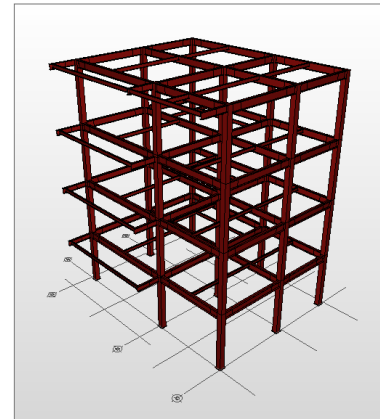
【(全階) 柱・梁以外の部材を OFF にした例】
