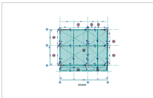
【R階 梁伏図】
