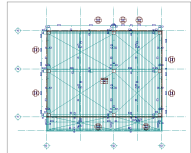
【4 階：完成図】
