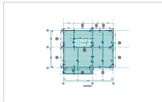
【4階 梁伏図】
