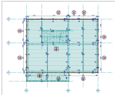
【2 階：完成図】
