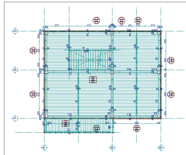
【3 階：完成図】
