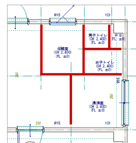
【LGS 壁を配置する箇所】
