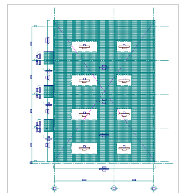
【バルコニーー東 4 階】
