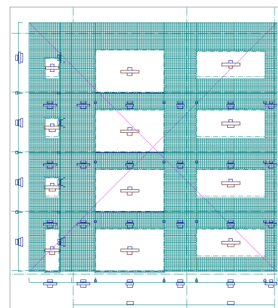
【南 B 4 階（伸縮目地）】
