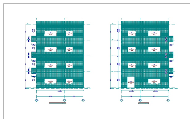
【タイル割付図（立面－東・西面）】
