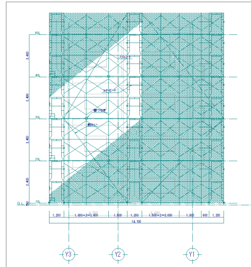
【立面図－西面】
