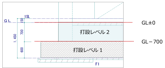
【基礎断面図】
