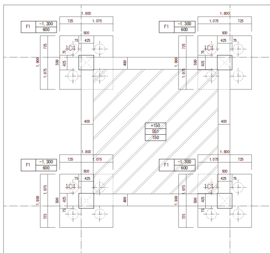
【基礎伏図】
