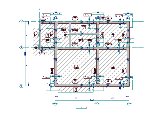
【底盤伏図】
