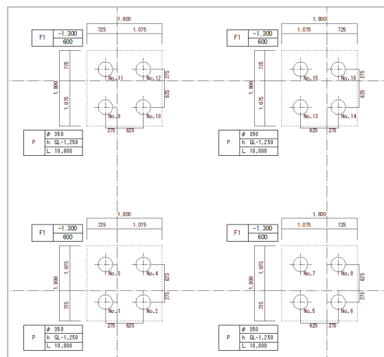
【杭伏図】
