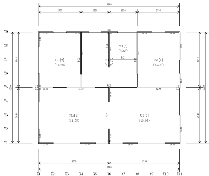
(2) 基礎反力図
