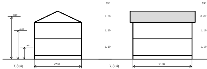
各階風圧力の算定（風力係数を考慮）
