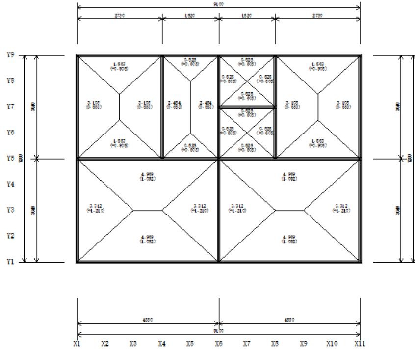
(1) 基礎梁負担図
