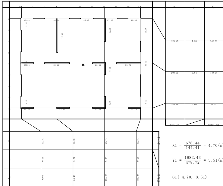
1階 重心図
