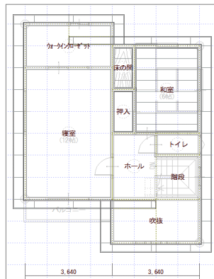
【2階 天井伏図】
