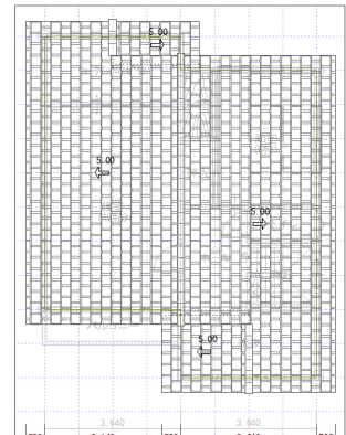
【2階 屋根伏図】
