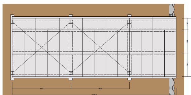
1F 構台伏図 1/50
