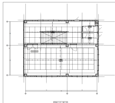
【天井インサート図】
