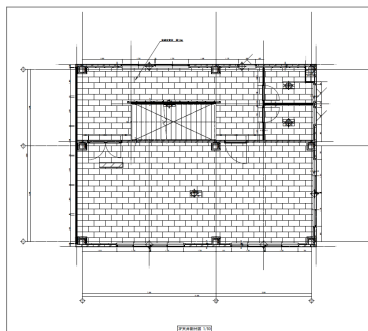
【天井割付図】
