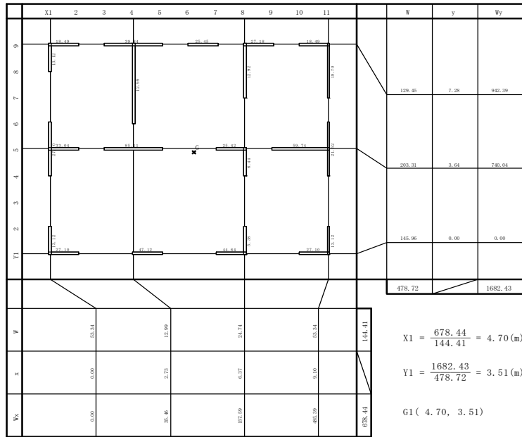
1階 重心図
