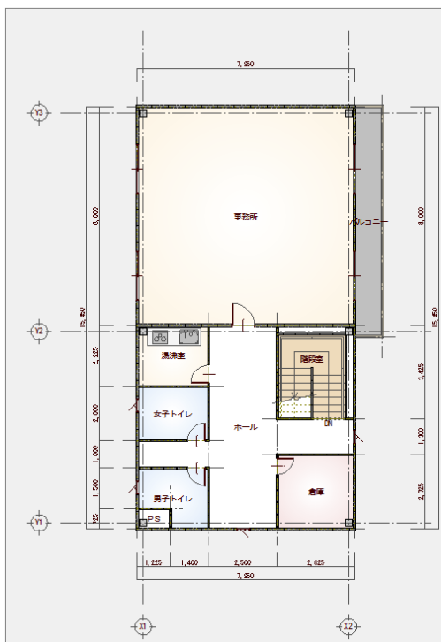
■ 3階 平面図
