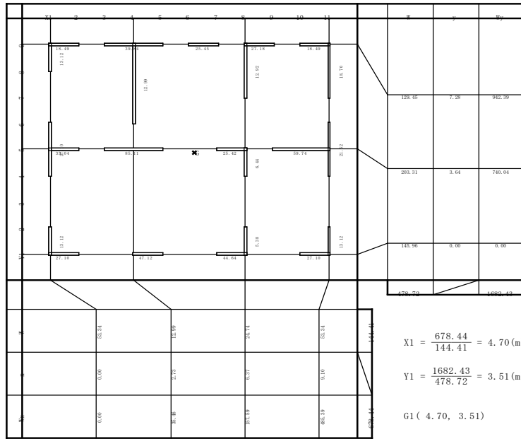
1階 重心図
