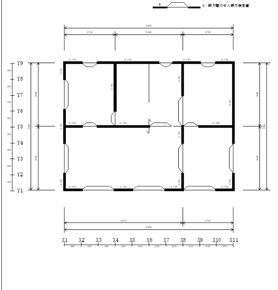
2階 短期荷重時検定比図
