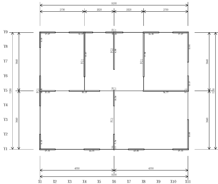
基礎略伏図及び軸力
