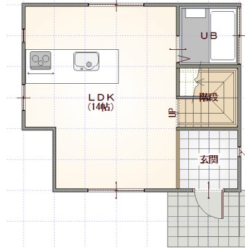
【1階 平面図】
