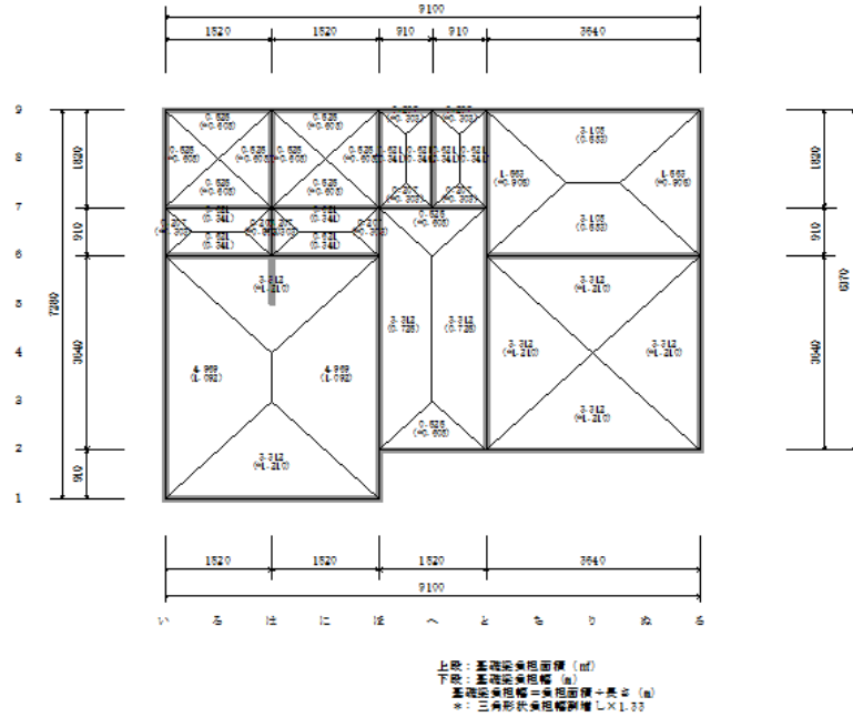
(1) 基礎梁負担図
