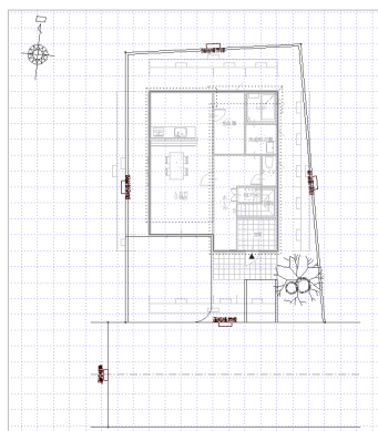
【配置図（2面）】
