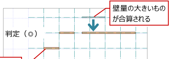
【図3：大きい壁量から合算】
