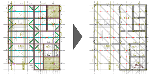
【1階 床伏図】
