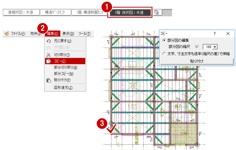
【1階 床伏図】
