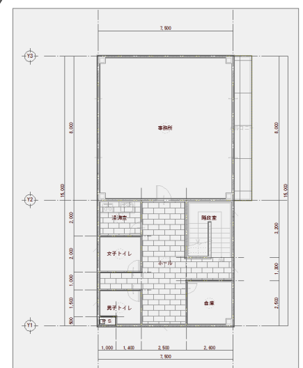
【3階天井伏図】
