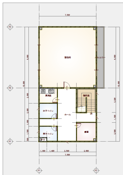
【3階平面図】
