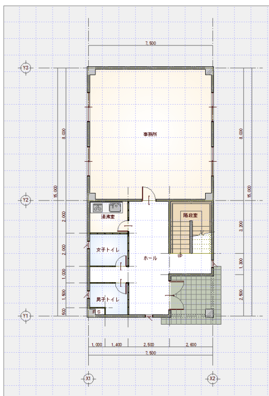
【1階 平面図】
