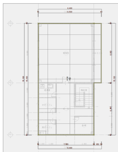
【3階屋根伏図】
