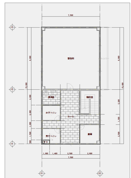
【3階天井伏図】
