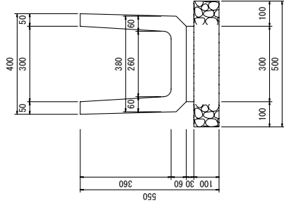
U型側溝 PU1型 1 : 10
