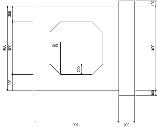
ボックスカルバート 1 : 20
