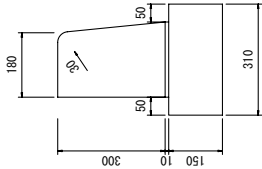
境界ブロック 1 : 10
